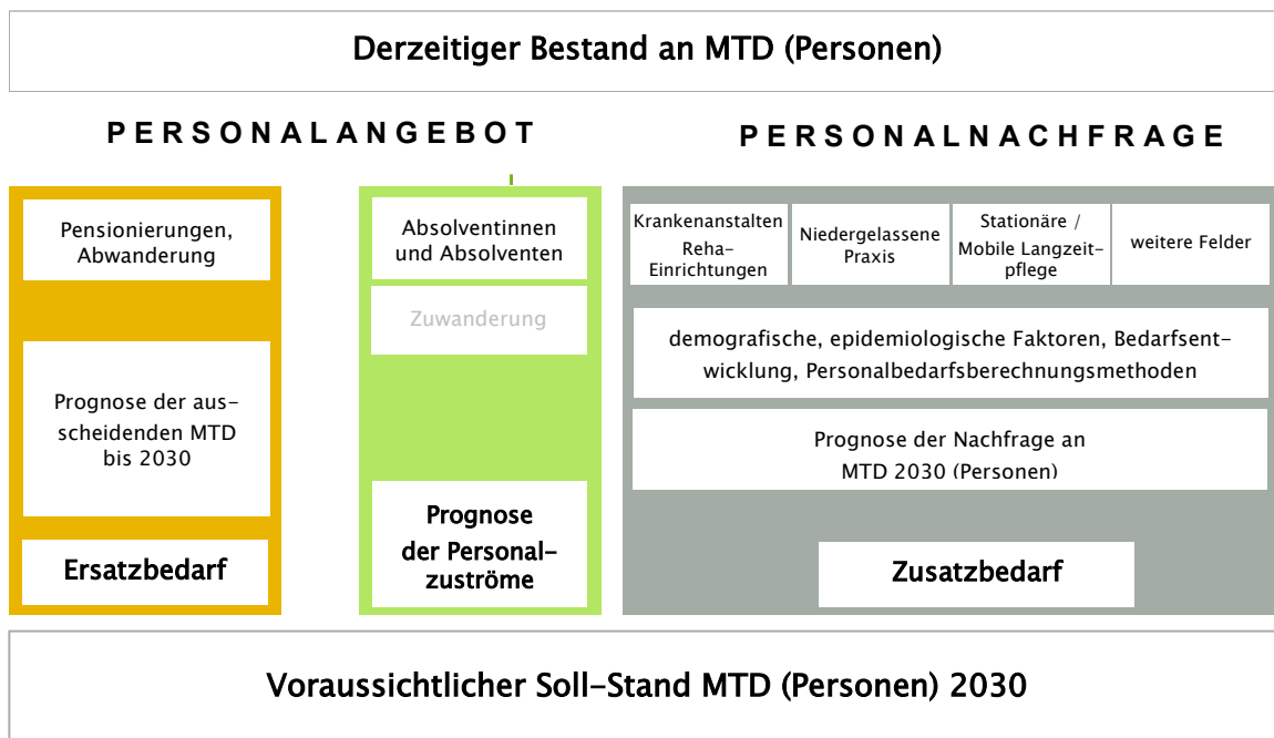
Abbildung 2.1: Prognosemodell
